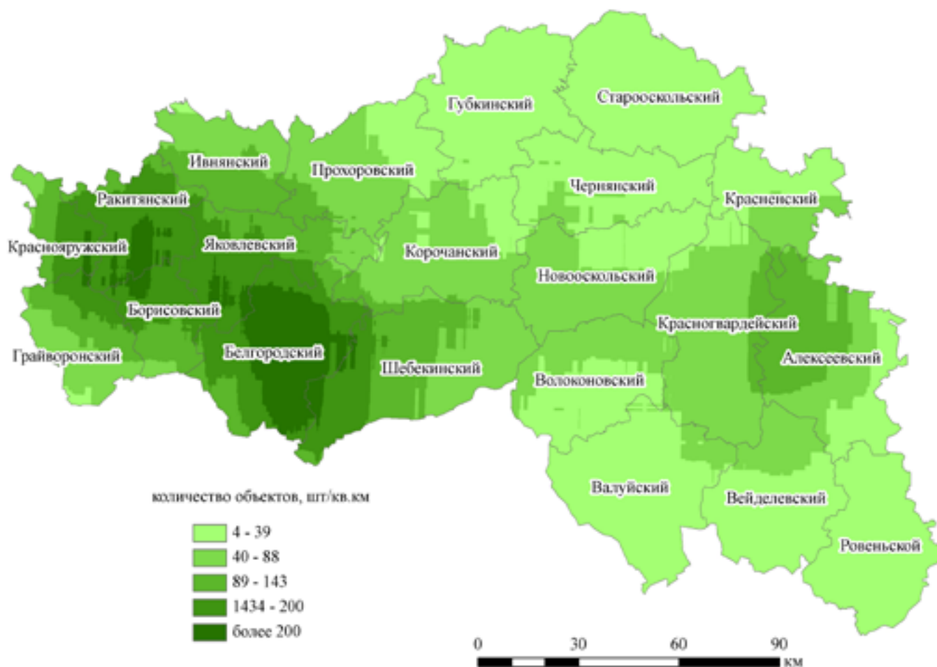
Рис. 1. Растровое моделирование плотности ООПТ в Белгородской области
